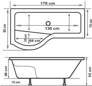
SW-5545 70 X 85 X 170 POLA OTURMALI
