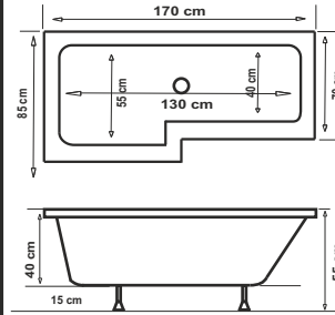
SW-5550 70 X 85 X 170 LOLA OTURMASIZ
