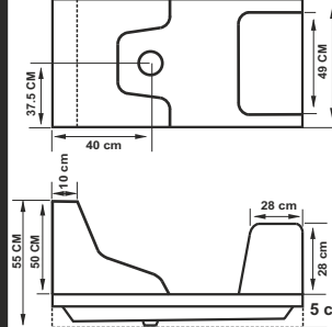
SW-5500 75 x 100 WELL KİŞİSEL BAKIM ÜNİTESİ 100 cm
