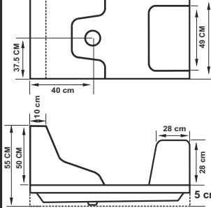
SW-5550 70 X 85 X 170 LOLA OTURMASIZ
