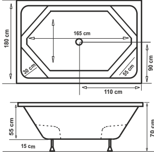
SW-5460 180 x 220 OPTİMUM ( KÖŞE OTURMALI ) 220 cm
