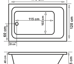
SW-5307 120*170 PECEFUL 170 cm
